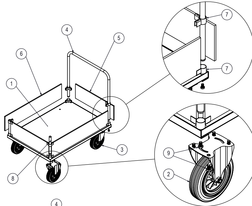
KMx35-xL
